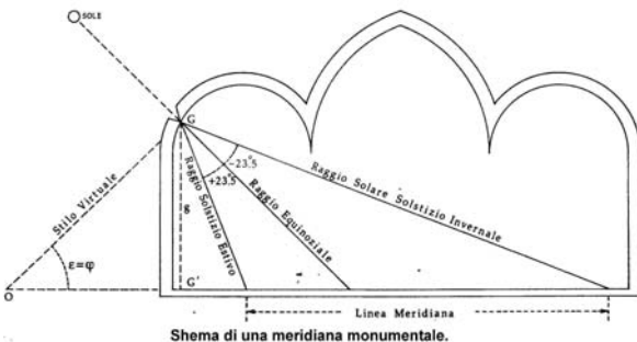
Nella meridiana "a camera oscura" il foro gnomonico rappresenta la punta di uno stilo polare virtuale (OG) il cui piede poggia sul prolungamento della linea meridiana.
